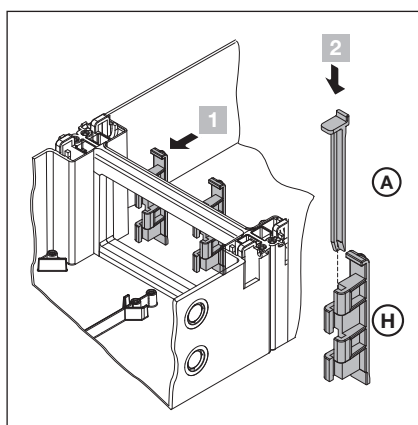
Abb. 3-16: Zusammenbau
