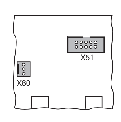
Abb. 7-16: X51 = Anschluss zur Steuerung, X80 = Anschluss für Zusatzplatten
