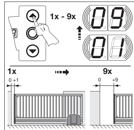
Abb. 6-24: Endlage Tor-Zu zurück Richtung Tor-Auf einstellen
