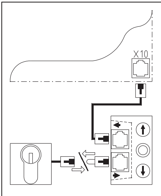
Abb. D/1 : Anschluß der Erweiterungen
