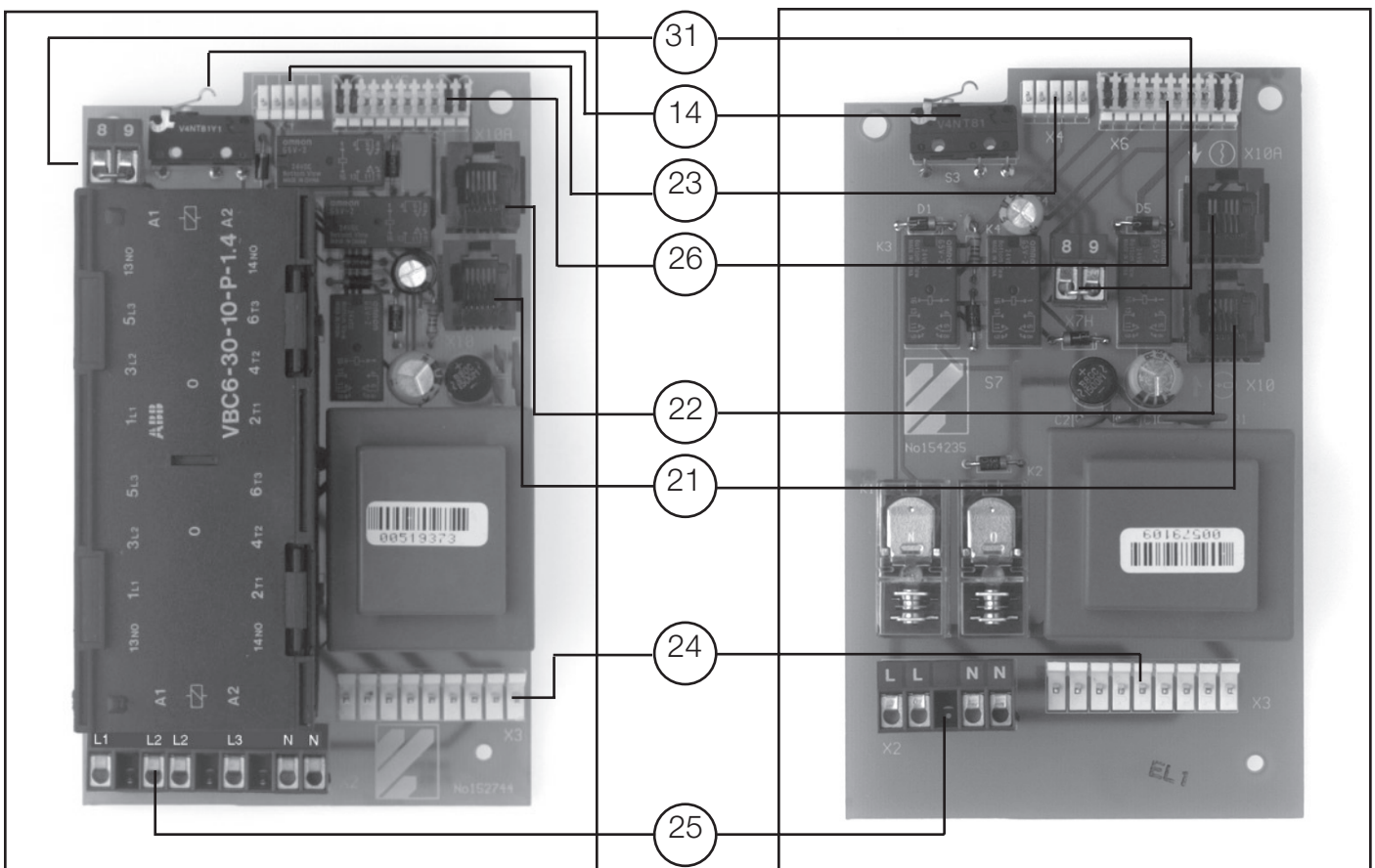
Abb. A/2: Steuerung A 40 N
