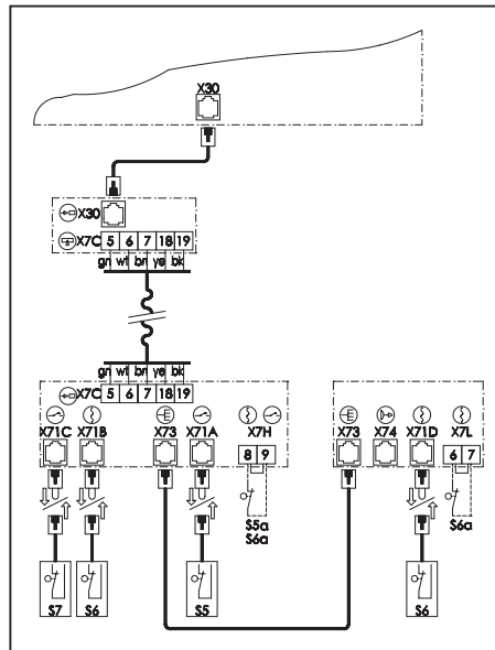
Abb. 4: Schaltplan
