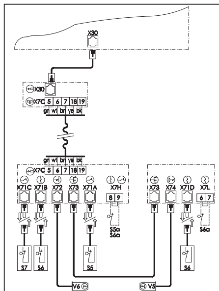
Abb. 7: Schaltplan
