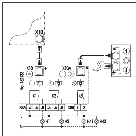
Abb. 12: Anschlussplan
