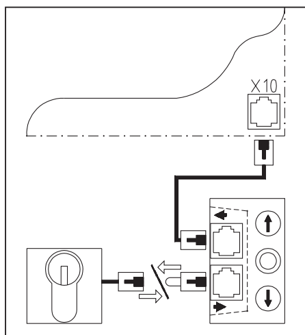
Abb. 9: Schaltplan
