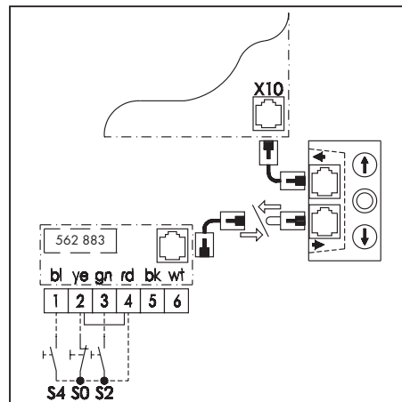
Abb. 10: Anschlussplan
