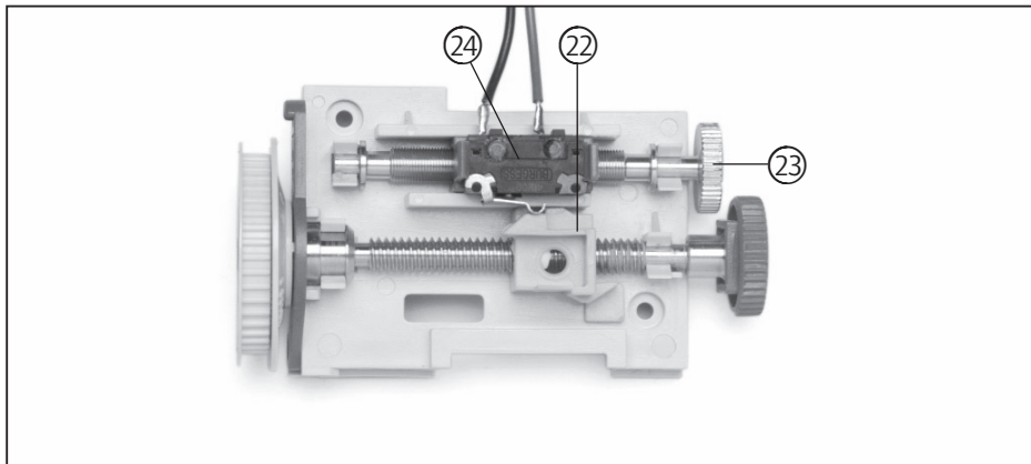
Abb. 6: Referenzpunkteinstellung (Tor ist geöffnet)
