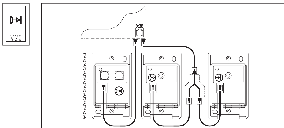
Abb. 11: Schaltplan
