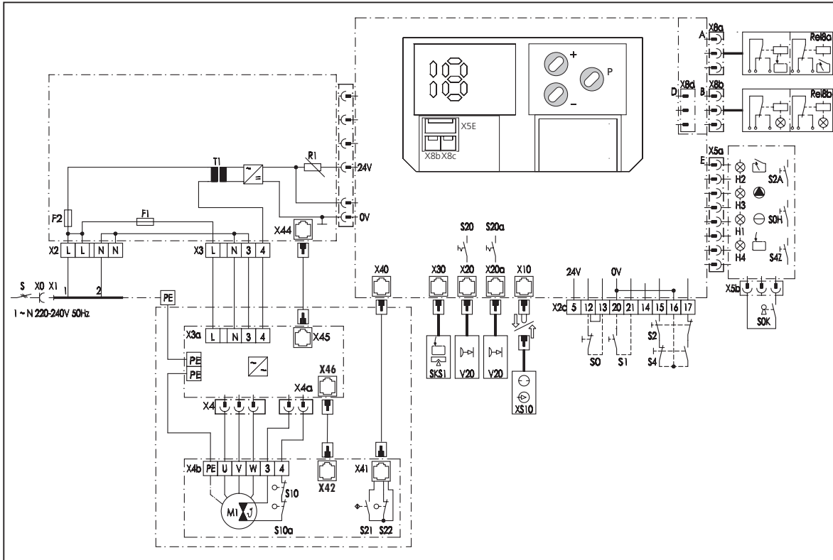
Abb. 28: Schaltplan
