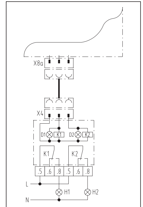
Abb. 22: Schaltplan
