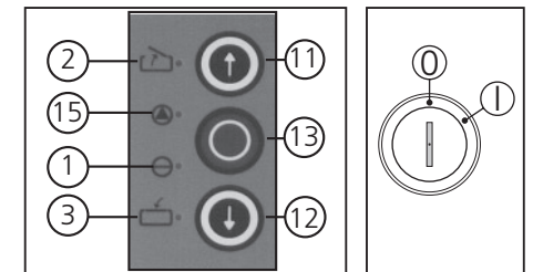
Abb.2: Folientastatur und Schlüsselschalter
