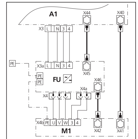
Abb. 10: Schaltplan
