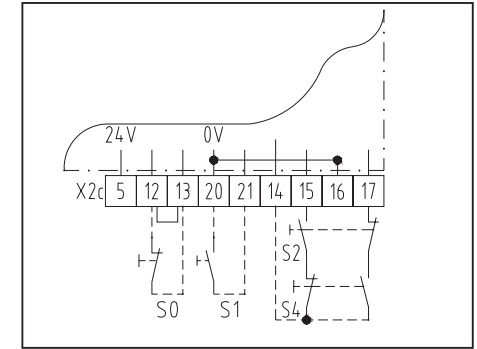
Abb. 20: Schaltplan
