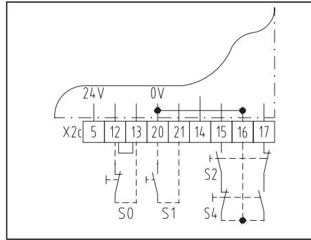
Abb. 18: Schaltplan
