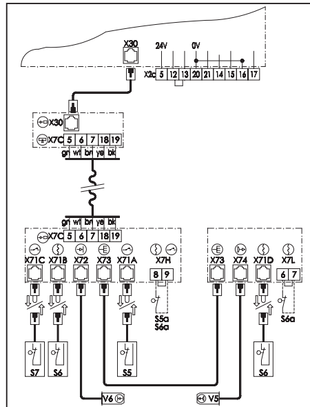
Abb. 15: Schaltplan
