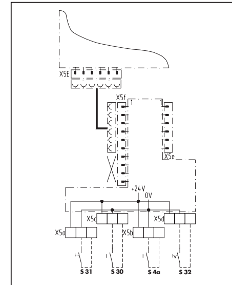
Abb. 26: Schaltplan
