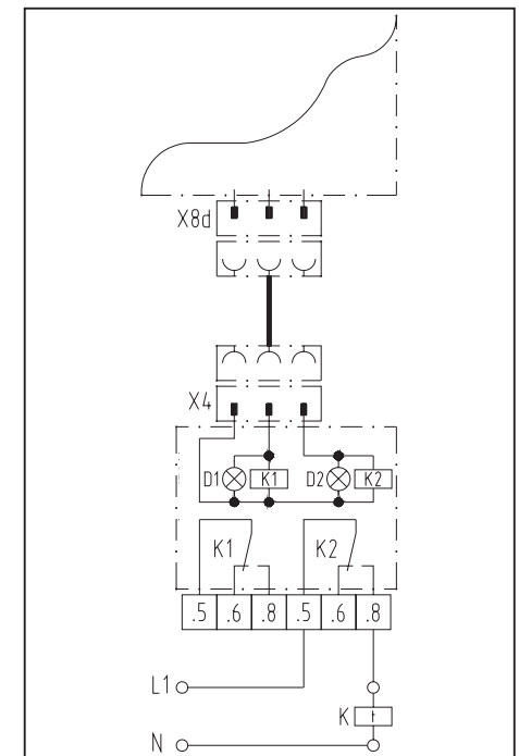
Abb. 27: Schaltplan
