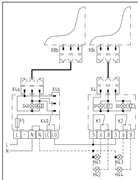
Abb. 25: Schaltplan
