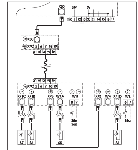
Abb. 11: Schaltplan
