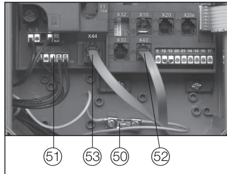
Abb. 8: Anschlüsse in der Steuerung B 60 FU
