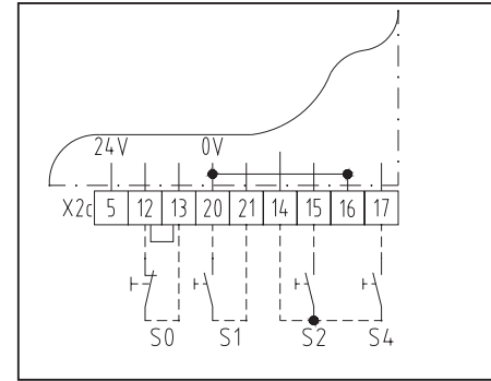
Abb. 19: Schaltplan
