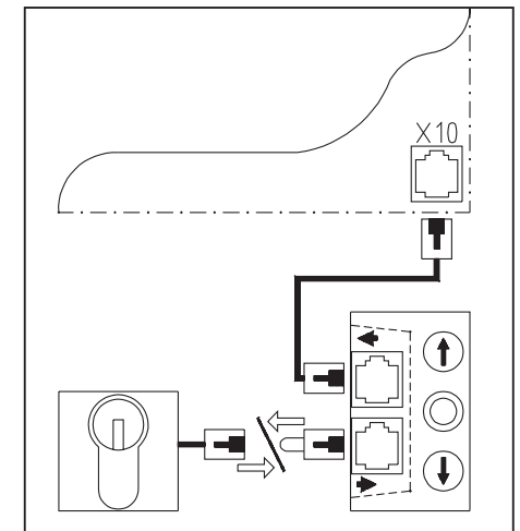
Abb. 16: Schaltplan
