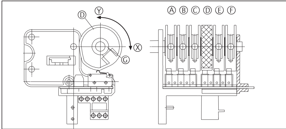
Abb. 14: SanftauslaufEinstellung Endlage AUF
