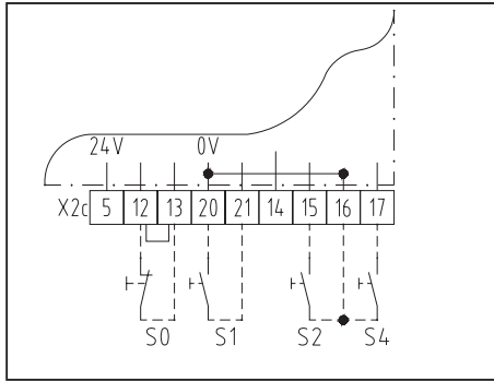
Abb. 17: Schaltplan
