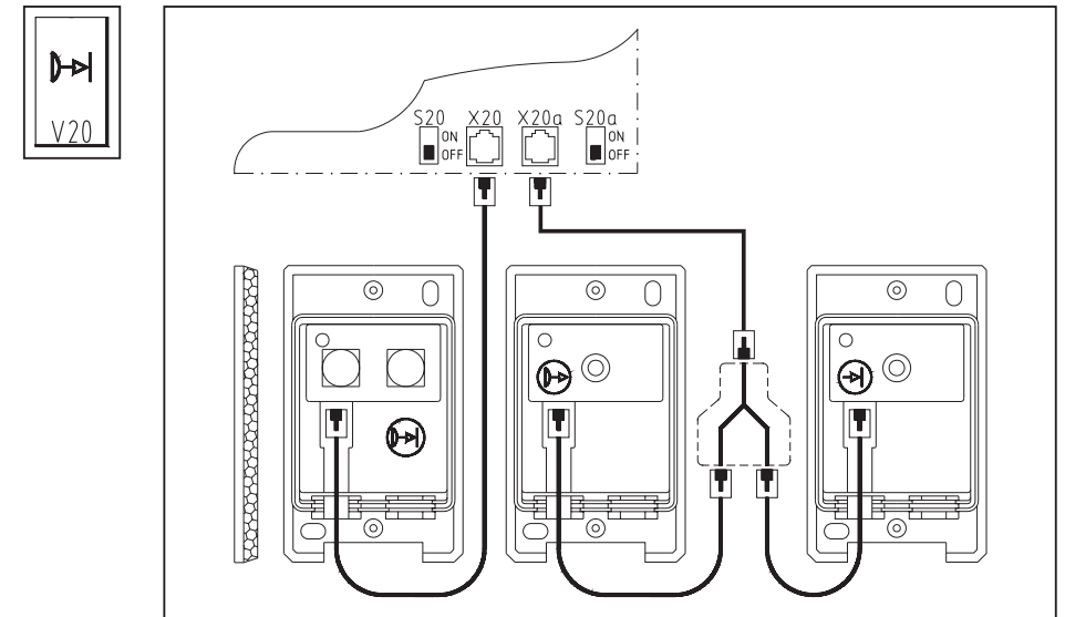
Abb. 21: Schaltplan
