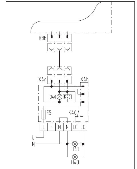
Abb. 23: Schaltplan
