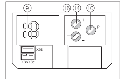
Abb.3: Bedienfläche der Steuerung
