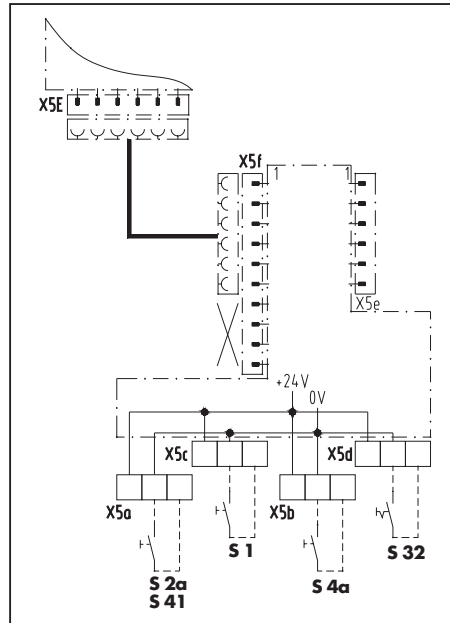
Abb. 24: Schaltplan
