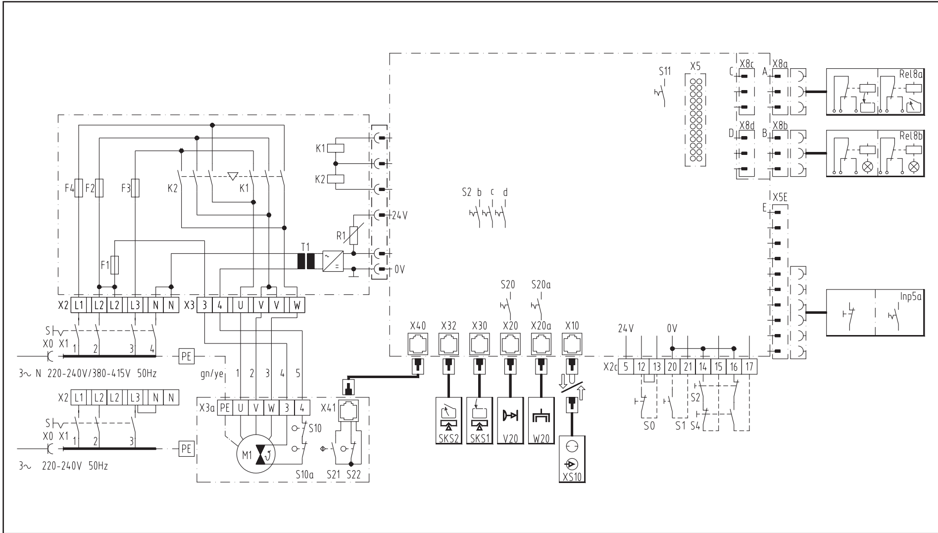
6.1.1 Schaltplan der Steuerung A 300
